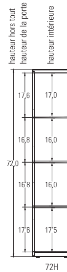
Quatre cases superposées GUTSS4
