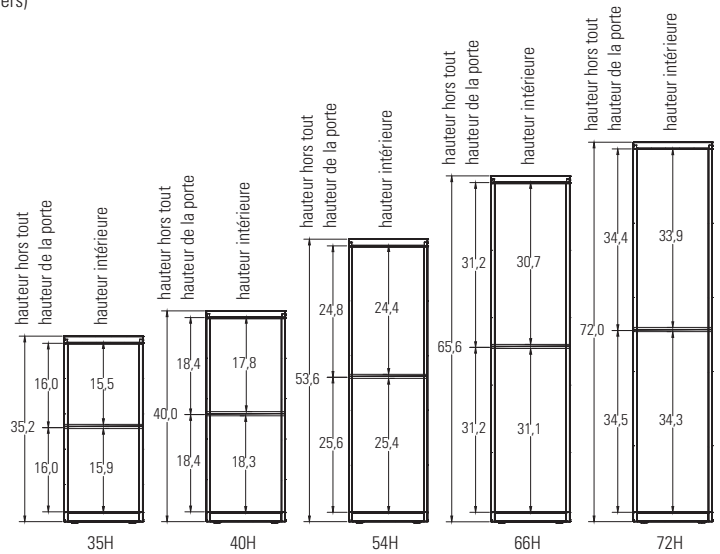
Deux cases superposées GUTSS2
