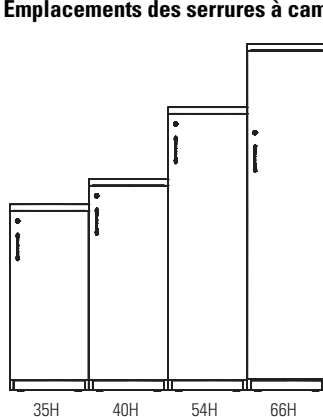
Une case GUTSS1
